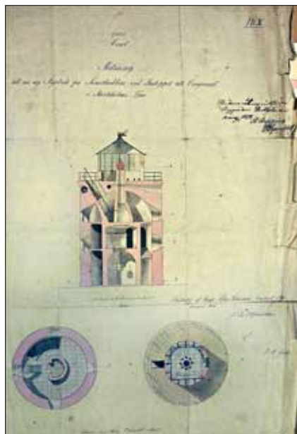
Svartklubbens fyr, ritning
